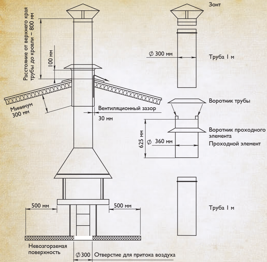
Принципиальная схема установки гриля LAPPIGRILL внутри беседок и террас
